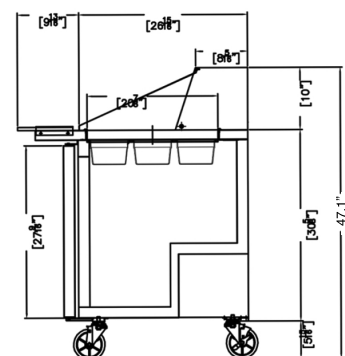
SIDE VIEW(1,2,3)
